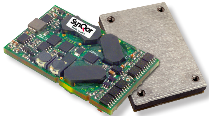
PQ40150QGx07 Module
